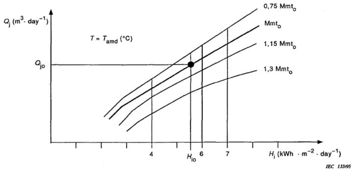
شکل ۱- آب دهی روزانه بر حسب تابش کل روزانه در سطح مدول
